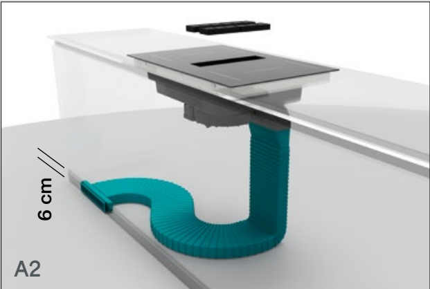
A2 KIT TUBI INSTALLAZIONE FILTRANTE ZOCCOLO H6 cod. 005PRC050001
