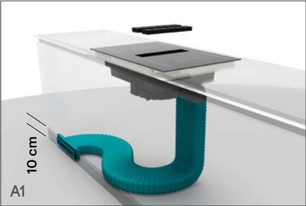
A1 KIT TUBI INSTALLAZIONE FILTRANTE ZOCCOLO H10 cod. 005PRC050002
