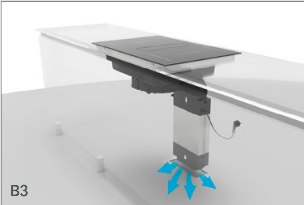
B3 INSTALLAZIONE FILTRANTE CON FILTRO AL PLASMA IN ARIA LIBERA (adatta anche per mobili con piedini)
