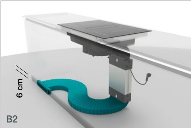
B2 KIT TUBI INSTALLAZIONE FILTRANTE ZOCCOLO H6 cod. 005PRC050001
